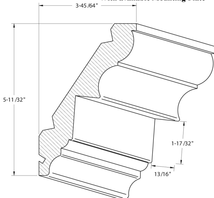
Crown 1623
