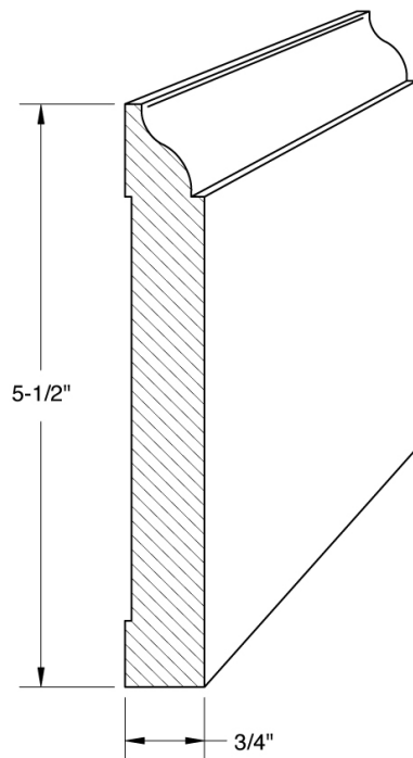
Base 898
