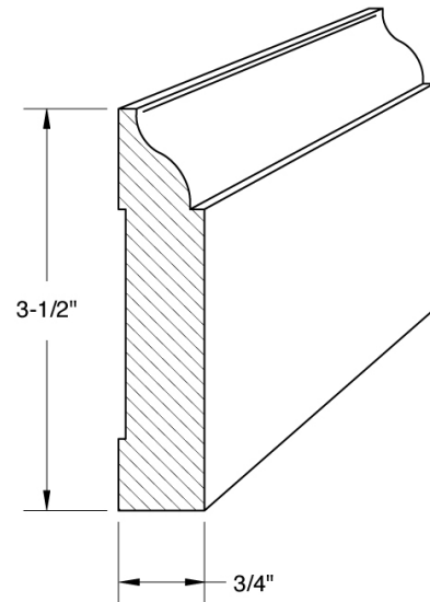
Base 897
