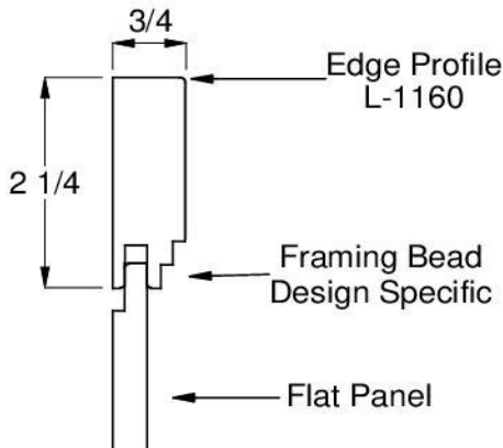
Edge Profile Option
