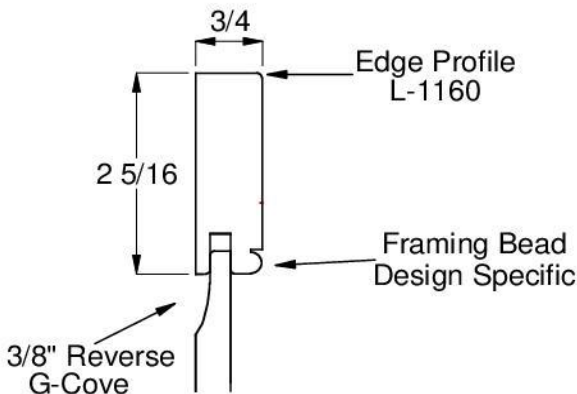
Edge Profile Option
