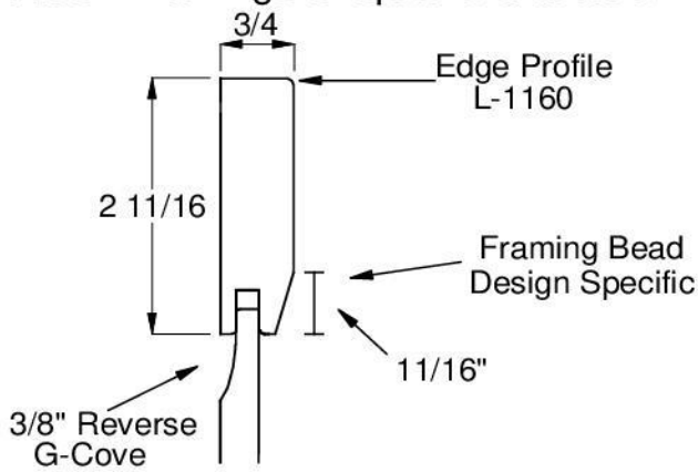
Door Panel Option
