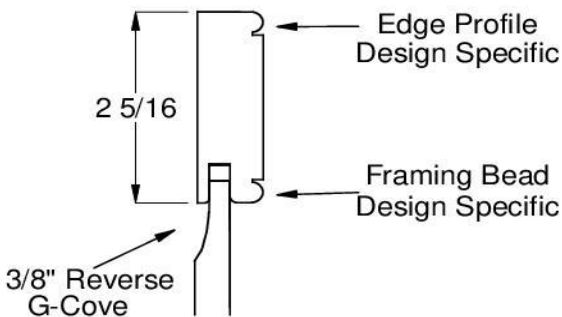
Door Panel Option
