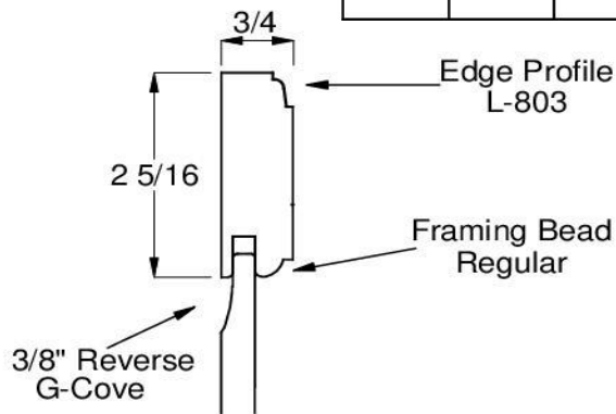
Door Panel Option
