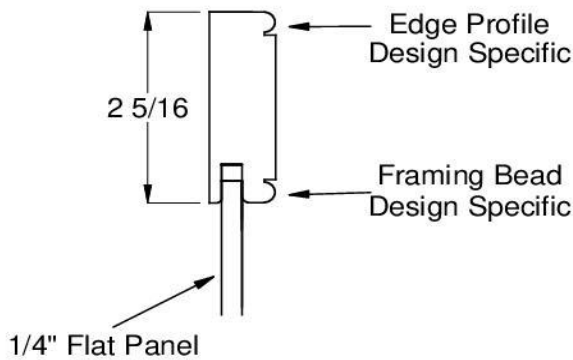
Door Panel Option
