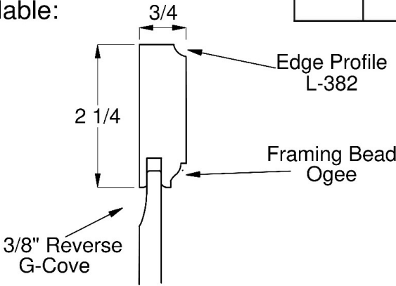
Door Panel Option
