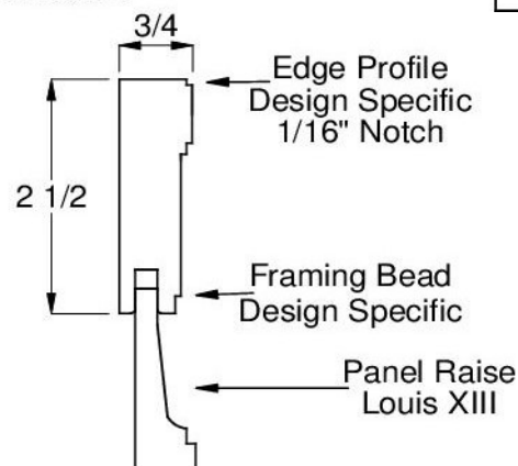
Door Panel Option
