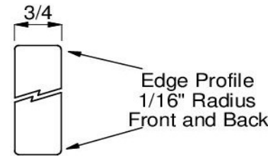
Door Edge Profile Option
