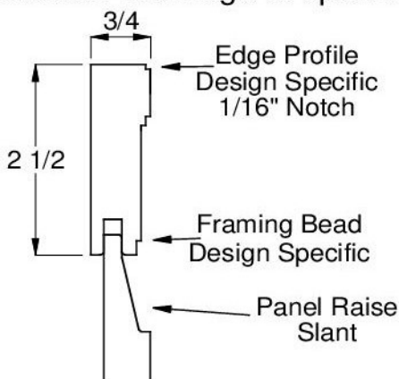
Door Panel Option
