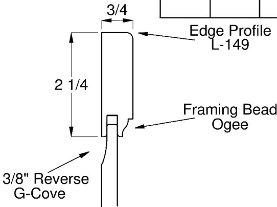
Door Panel Option
