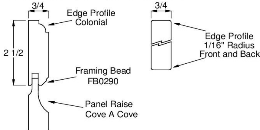
Door Edge Profile Option
