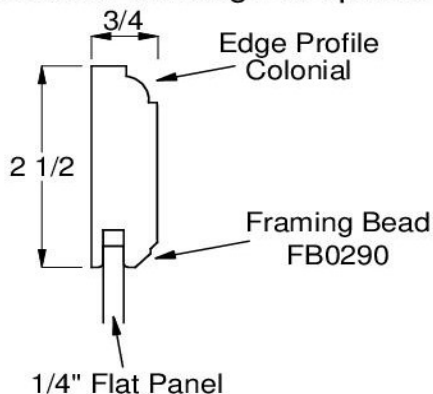
Door Edge Profile Option
