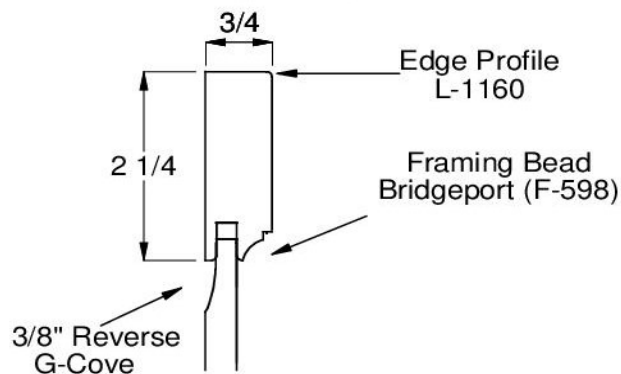
Door Panel Option
