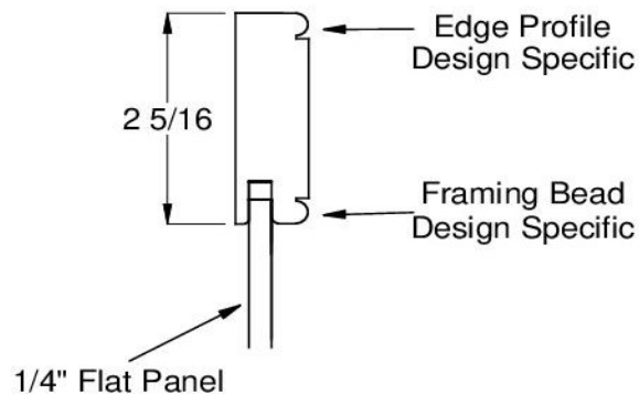
Door Panel Option
