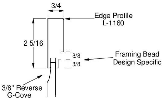
Door Edge Profile Option
