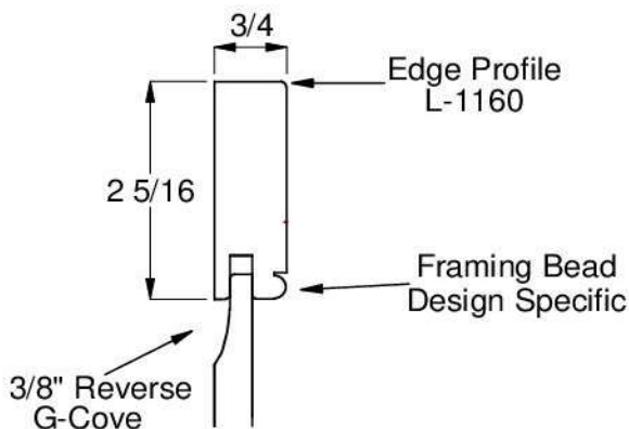
Edge Profile Option
